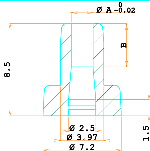
Sez. A-A
